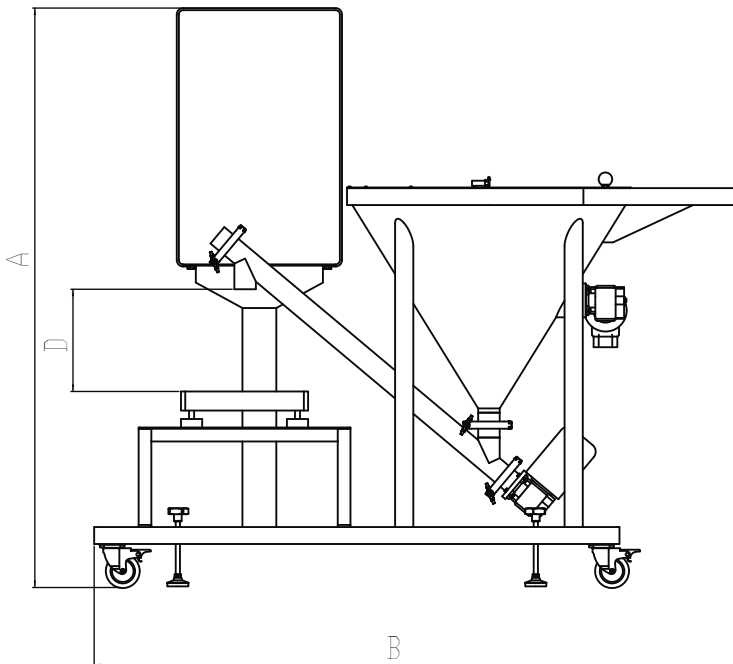
DMS Dosificador móvil para sólidos estándar
